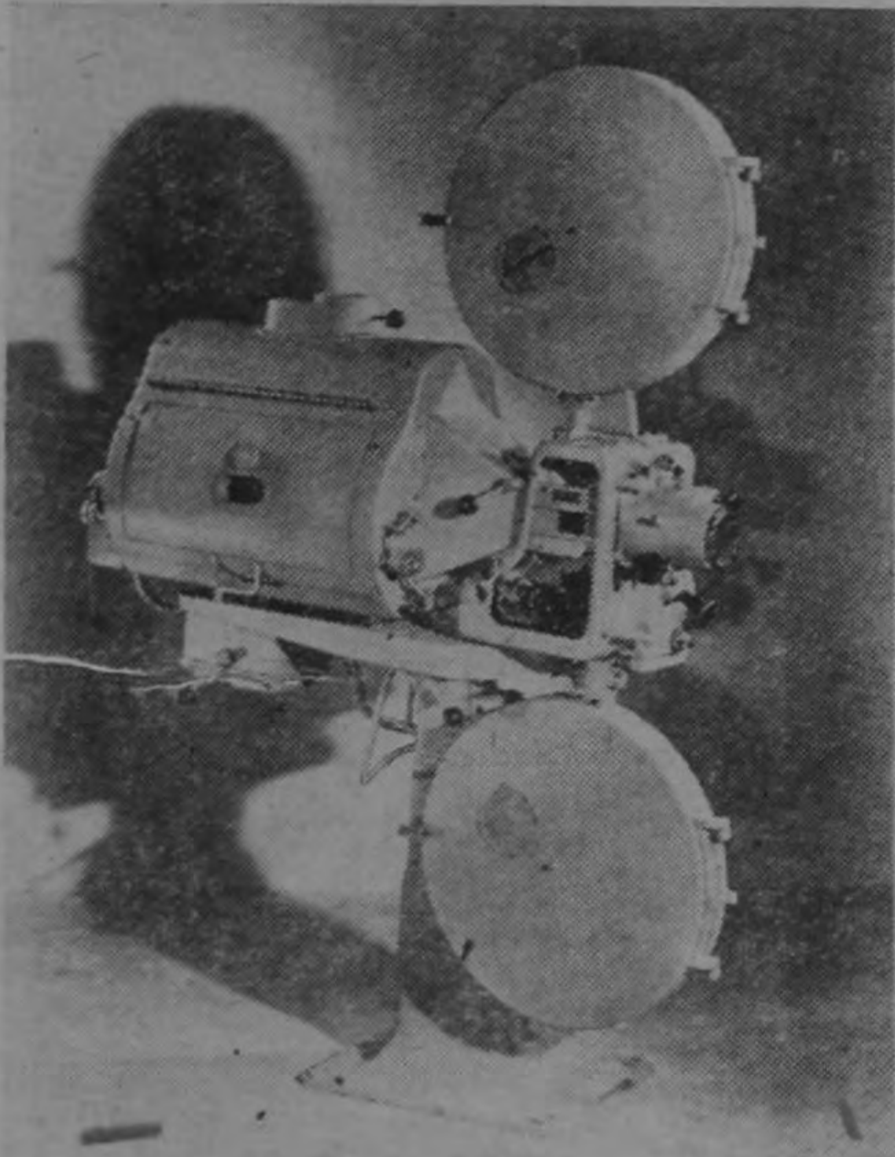
Proyector PHILIPS FP7 con refrigeración por agua, nuevo e ingenioso lector de sonido y máximo rendimiento luminoso.
